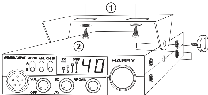
BEFESTIGUNG DES MONTAGEBÜGELS
